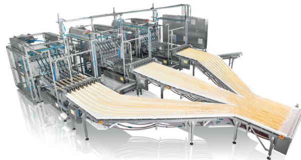
Série SCA Systèmes d'emballage de tuiles en tubes et/ou barquettes
