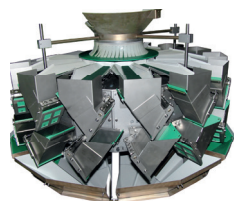
Série CP-HL (Heavy Load) Peseuses associatives pour charges lourdes
