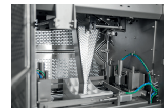
Systèmes de transfert Pour le remplissage de sachets, de boîtes, de barquettes etc.
